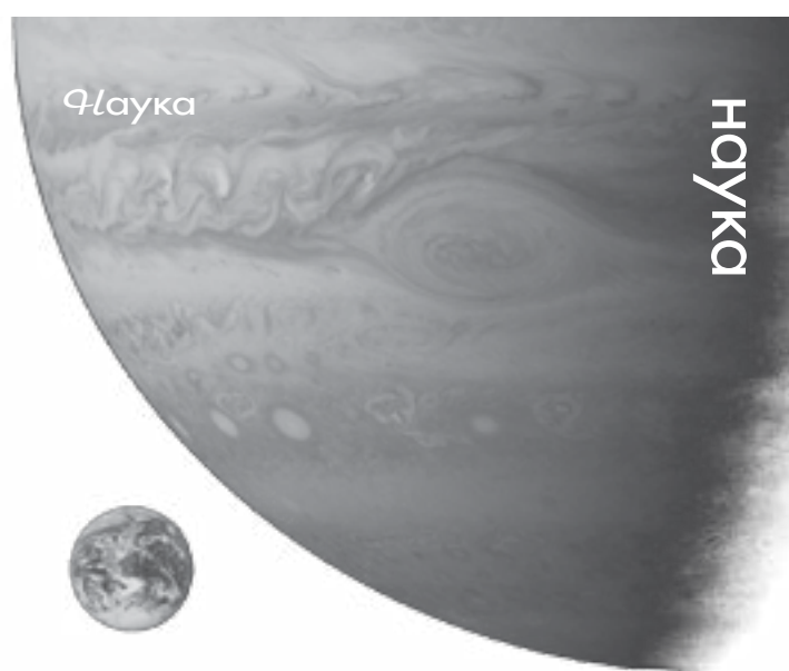
Юпитер и Земля [3]
