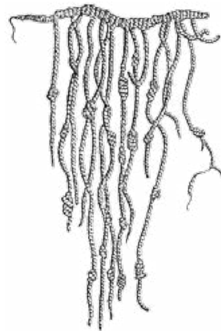
Счетное устройство инков.
